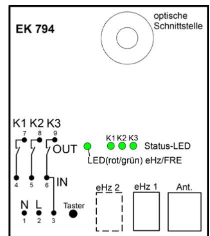
▲ EK794 - Funkrundsteuerempfänger Schaltbild
